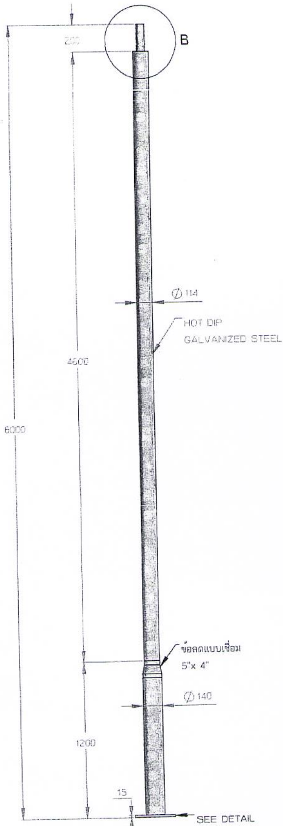
HI-WCS-060:เสาทกลมสูง6เมตรขนาด5นิ้วลด4นิ้ว SCALE 1 : 28
